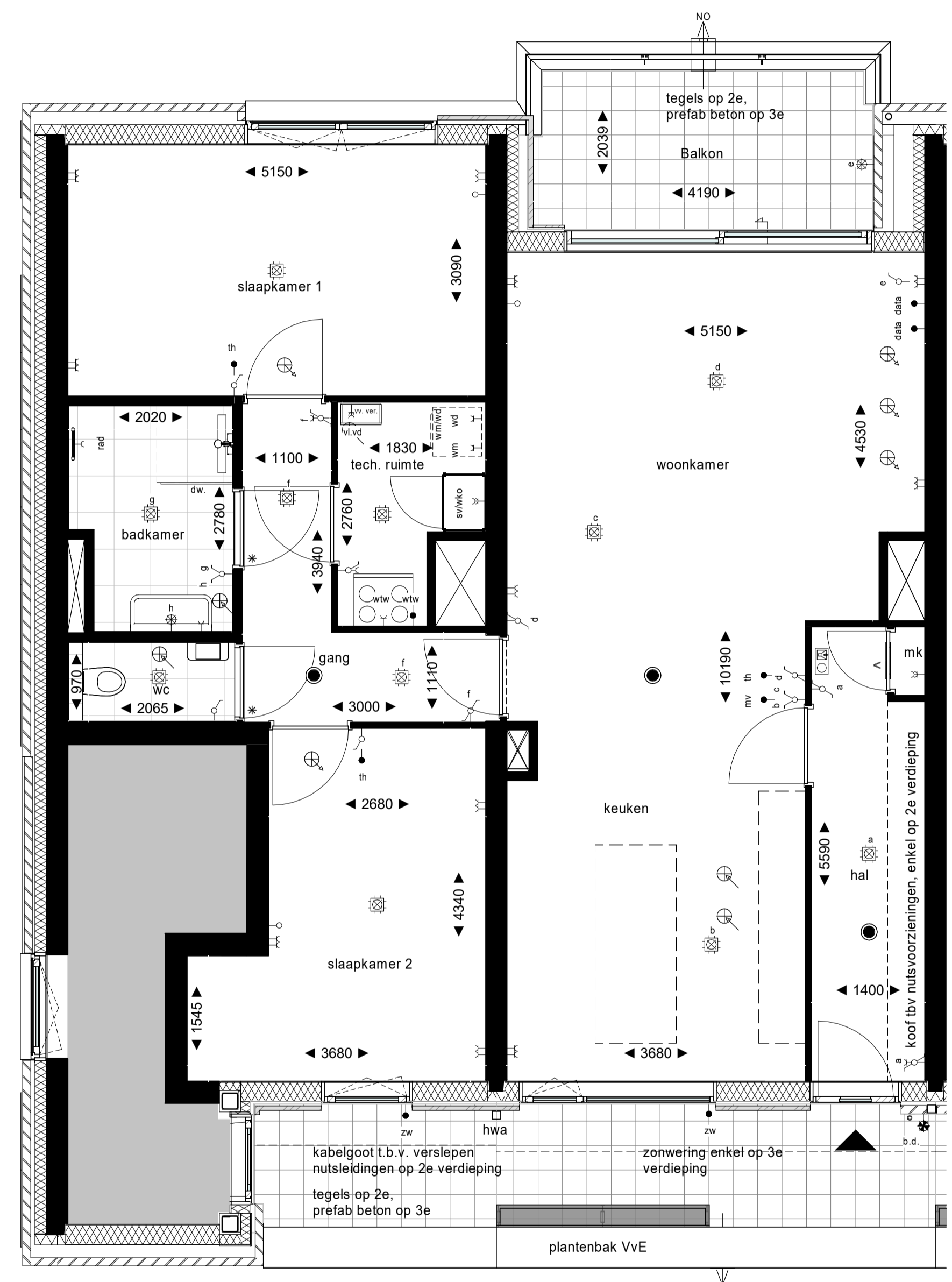
2e/3e verdieping
