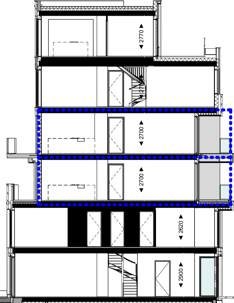
Doorsnede B-B
