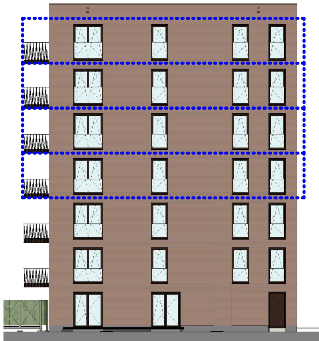
Noord-Westgevel 1 : 150
