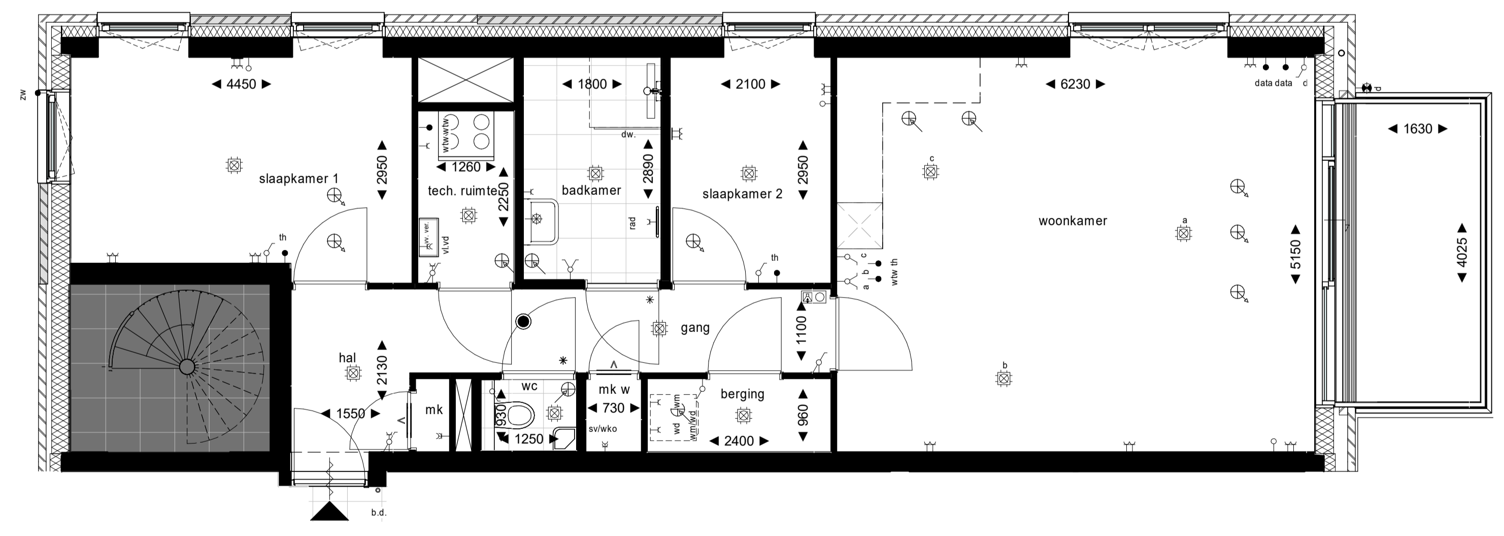
3e t/m 6e verdieping 1 : 50
