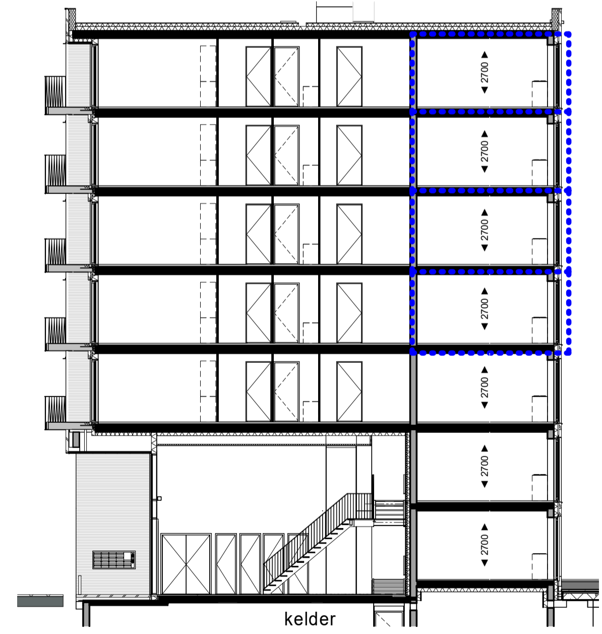
Doorsnede A-A 1 : 150
