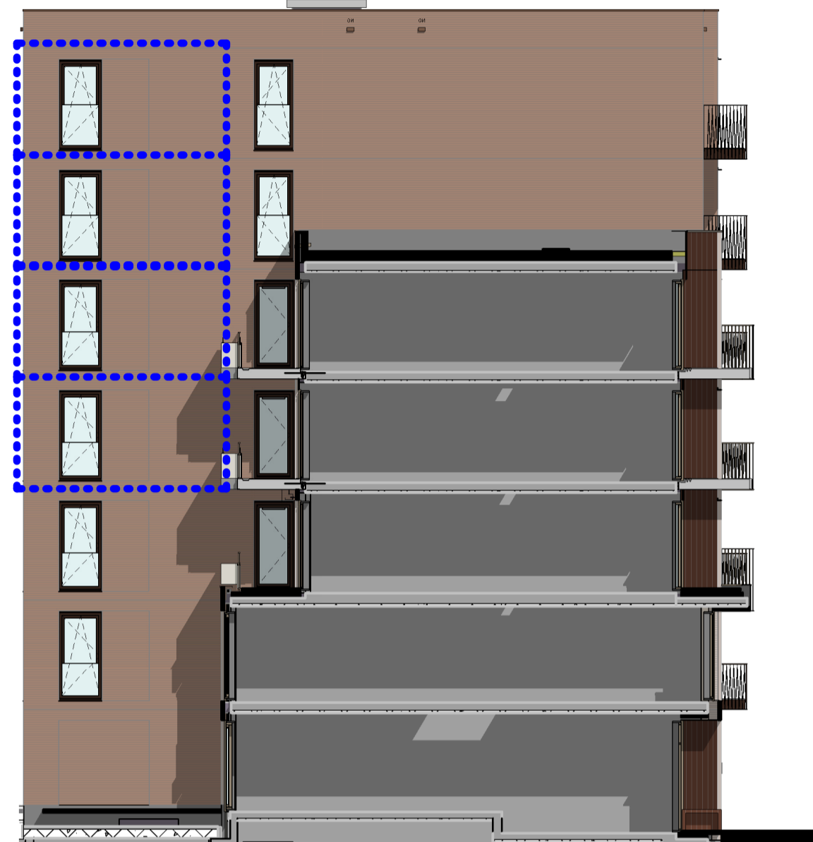
Zuid-Westgevel 1 : 150
